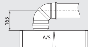
Dimna cev Ø 80/125
