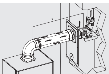
Vgradni sistem v obstoječo tuljavo Ø 60 do 13 m ali Ø 80
